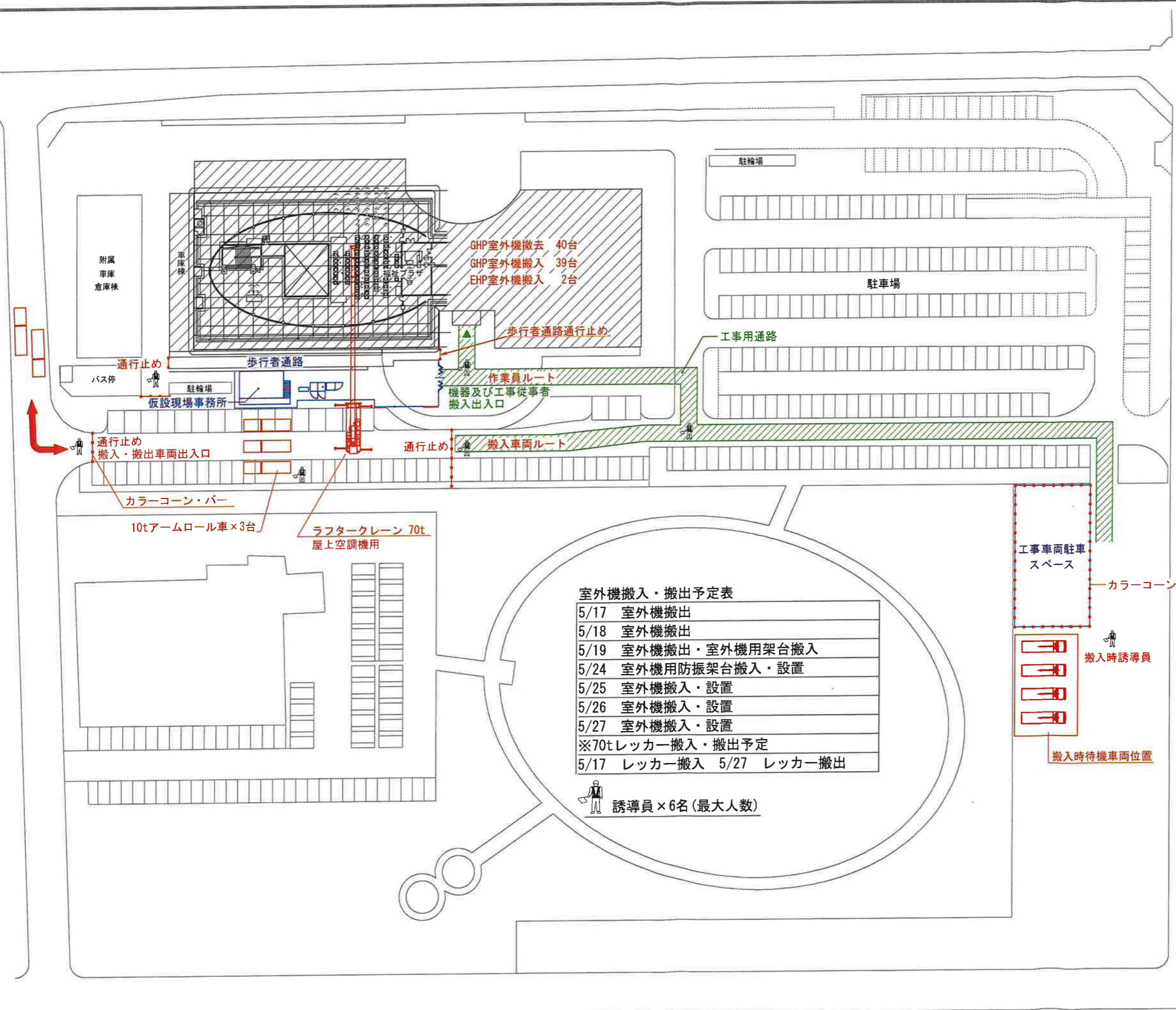
撤去・搬入計画図
